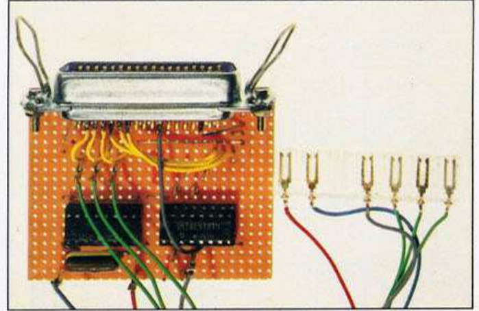
Bild 6. Nur wenige Bauteile werden für den Multiplexer Typ 3 gebraucht
